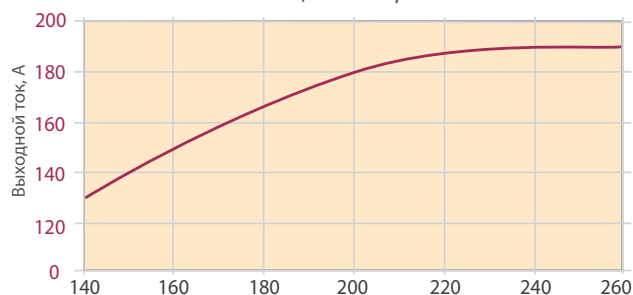
Зависимость величины максимального выходного тока от величины питающего напряжения
